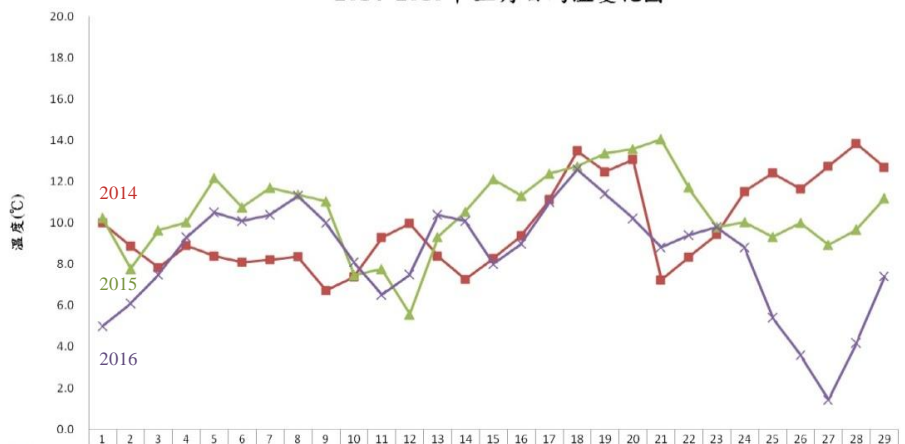
2014~2016年三月日均溫變化圖
